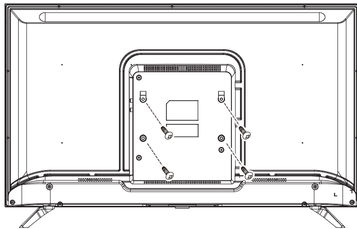
取り付けネジM6×12mm×4本
