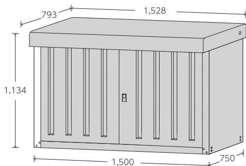
DSLB-1511
