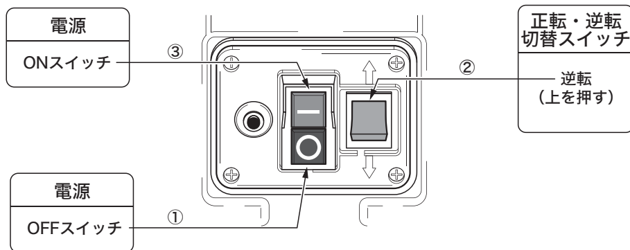
スイッチ説明図 ローラーミル刃の逆転
